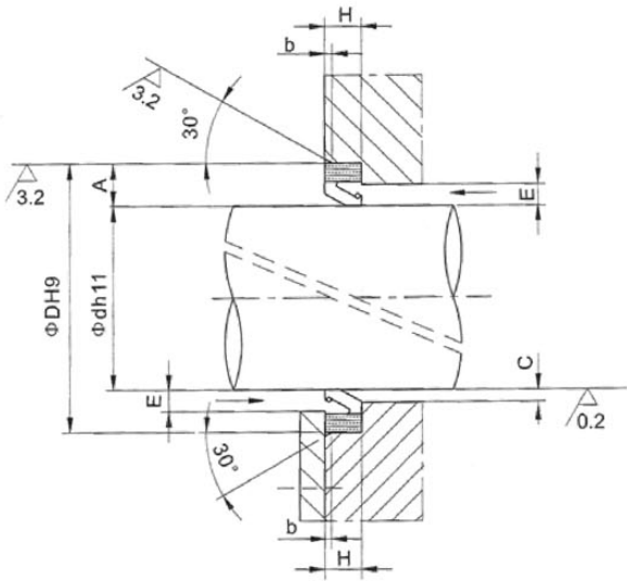
B 无涵盖压紧的结构式Carcoseal/SF
