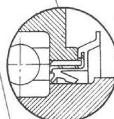
REAR AXLE 后轮轴用油封 KCY 型
