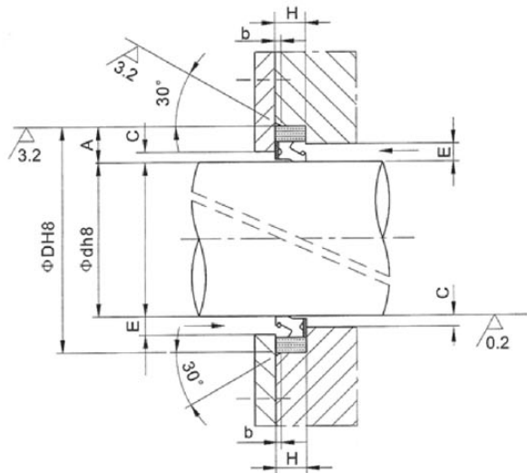
普通耐压旋转油封 Carcoseal/AP
