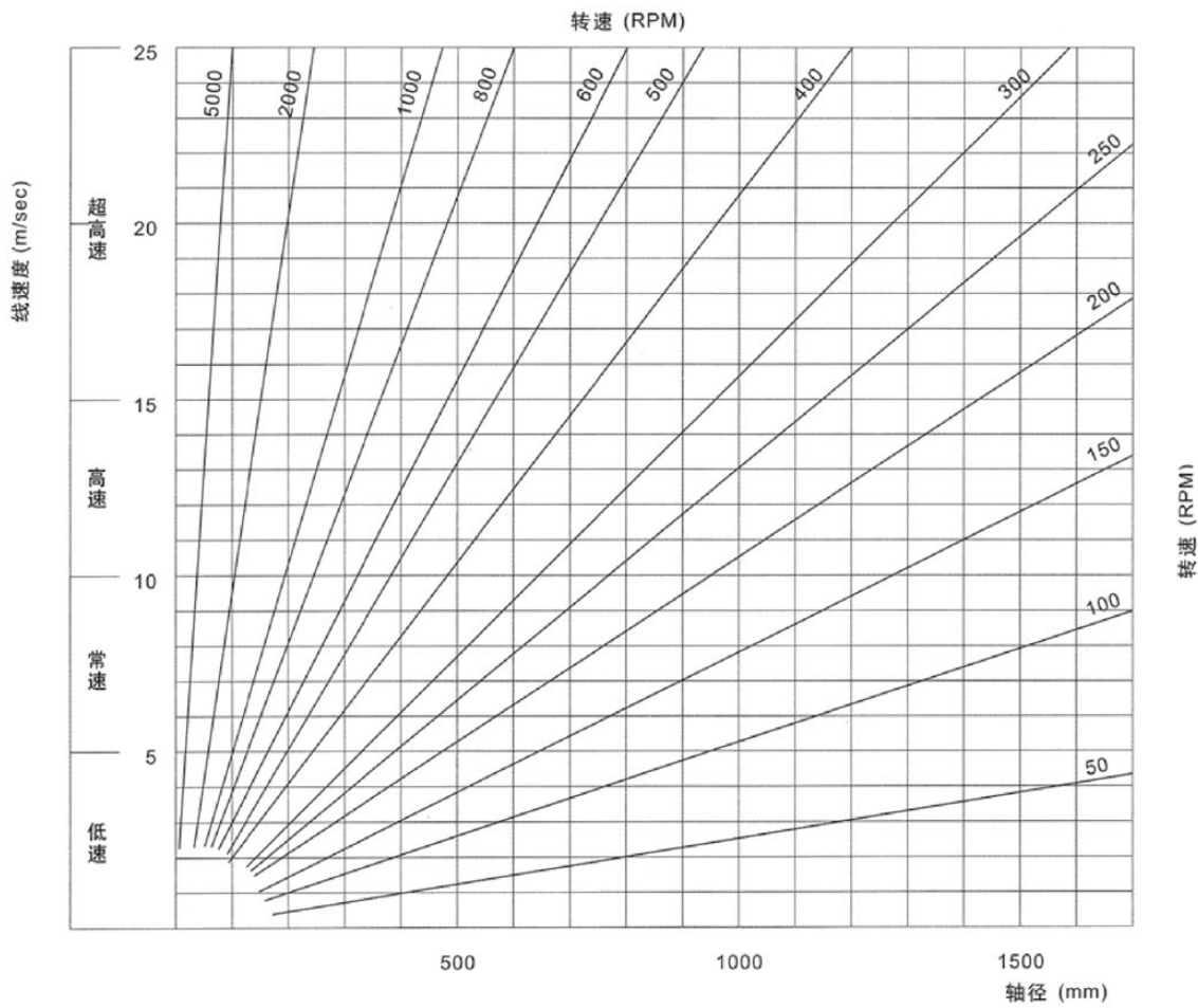
转速与线速度转换表
