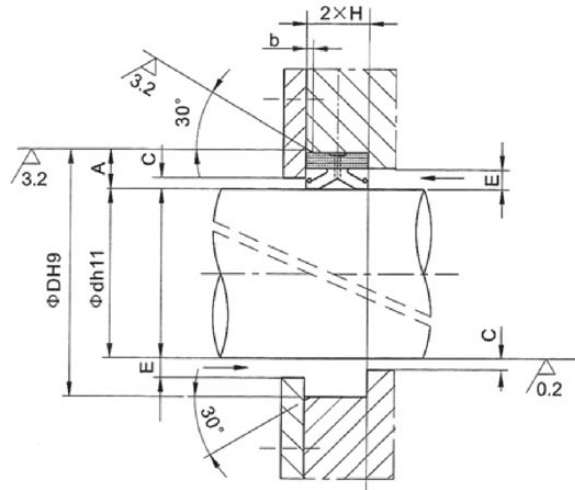
开口式加润滑油旋转油封
