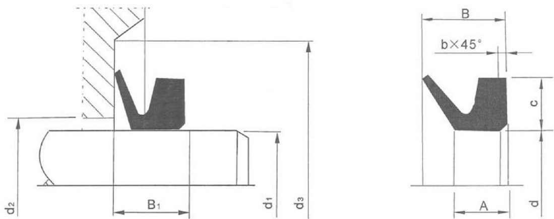
VE型V形环安装图及尺寸表
