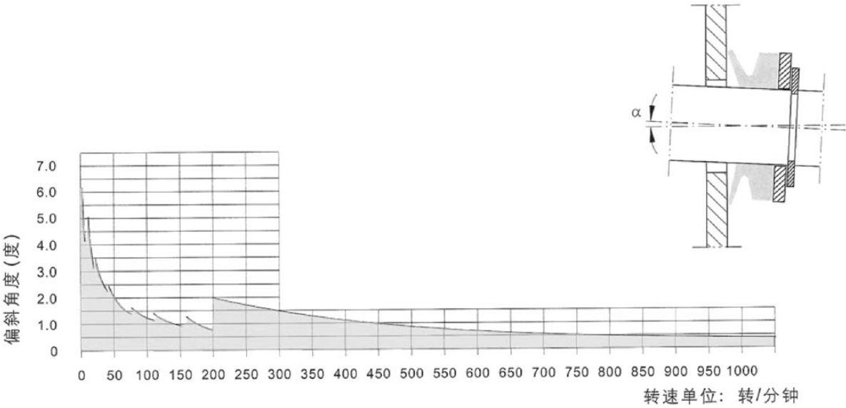
图表1 VA和VS型V形环设计上允许的最大偏斜角度
