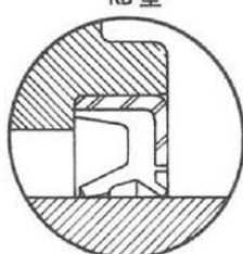
方向盘组件用油封 KB 型
