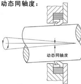
动态同轴度：
