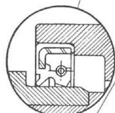
ENGINE FRONT 发动机曲轴用油封 (前)
