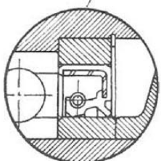
ENGINE REAR 发动机曲轴用油封 (后)
