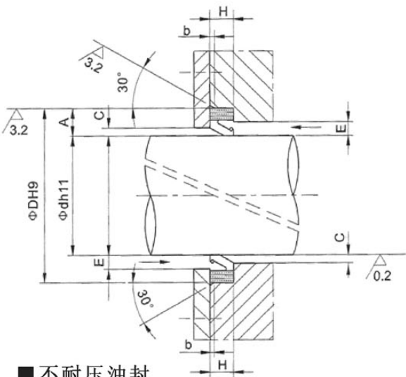
■ 不耐压油封
